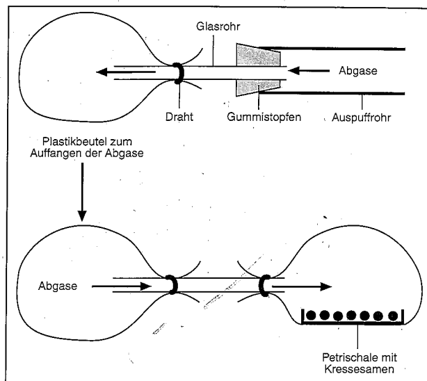
Versuchsaufbau
